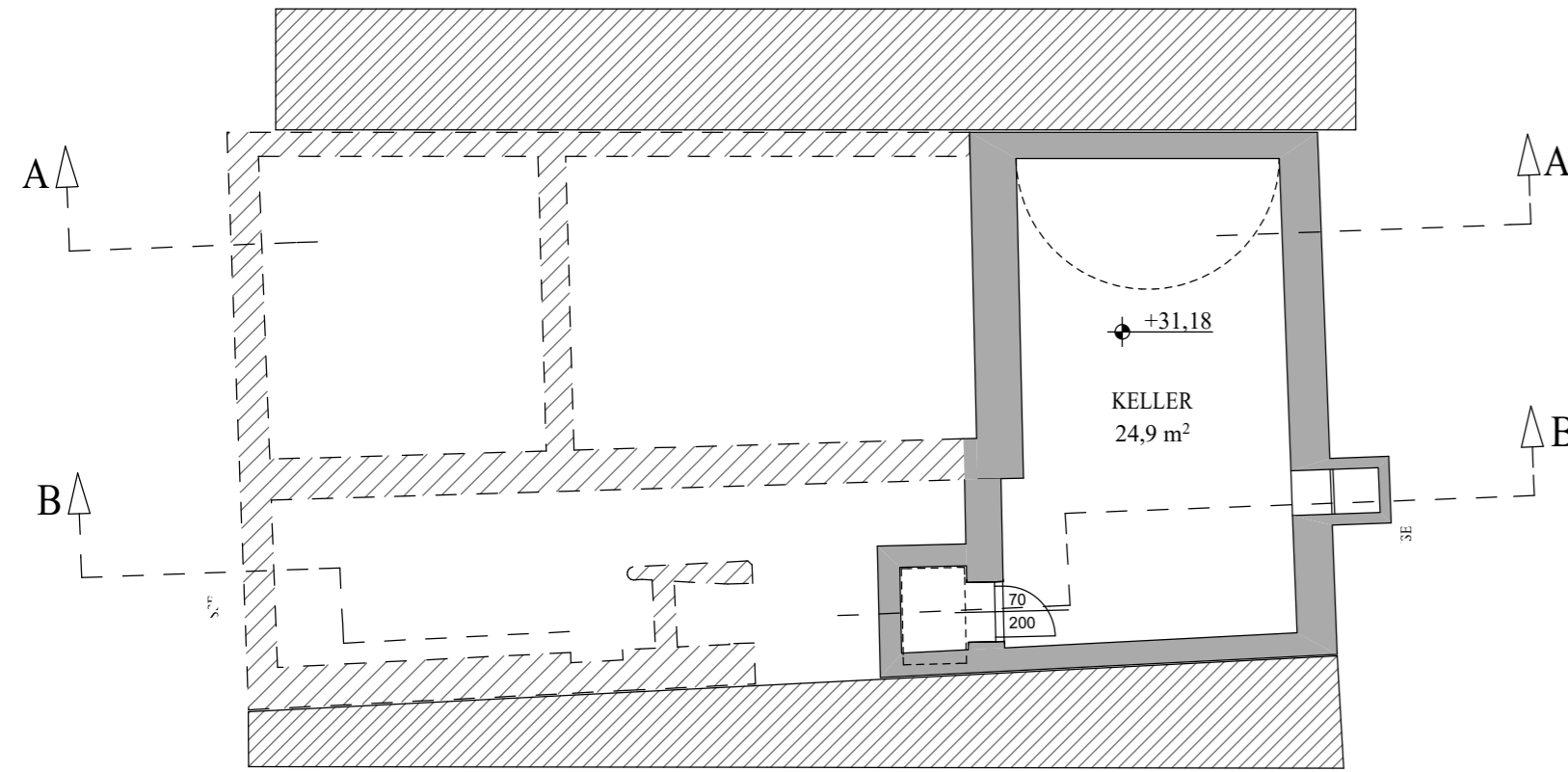
KELLERGESCHOSS 1:100
