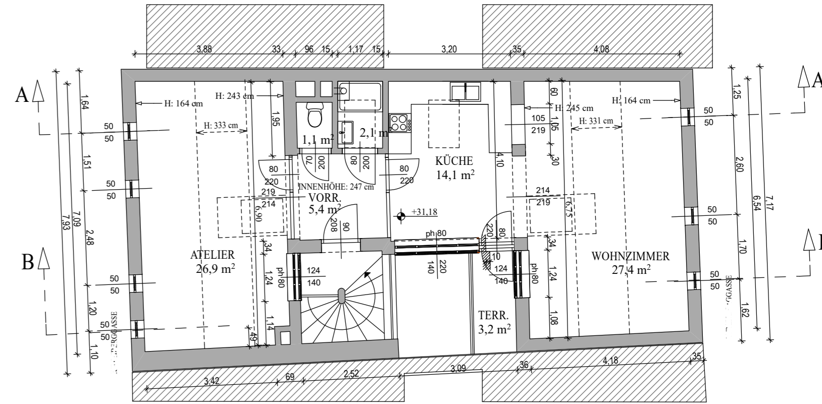
DACHGESCHOSS 1:100
