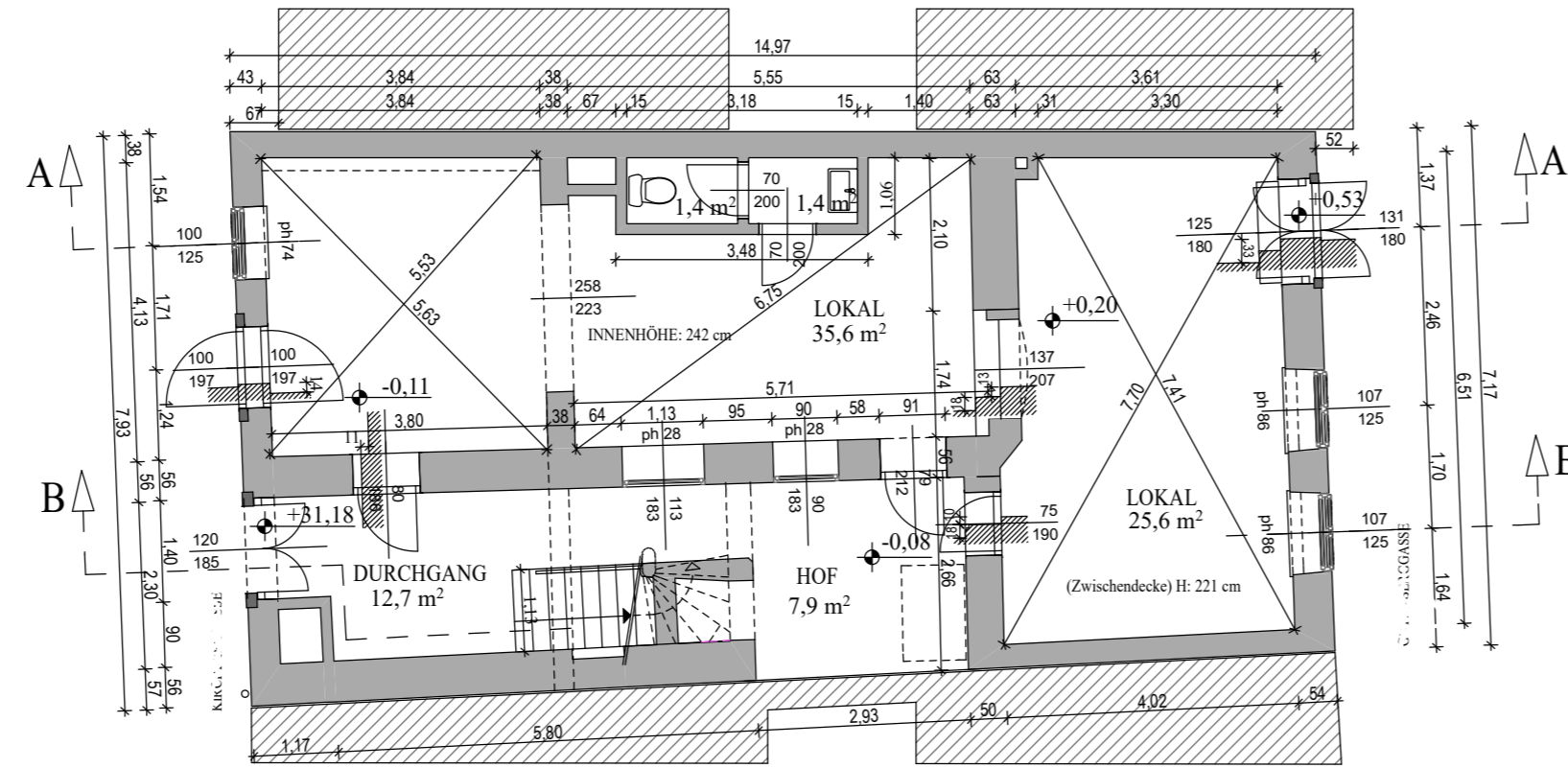
ERDGESCHOSS 1:100
