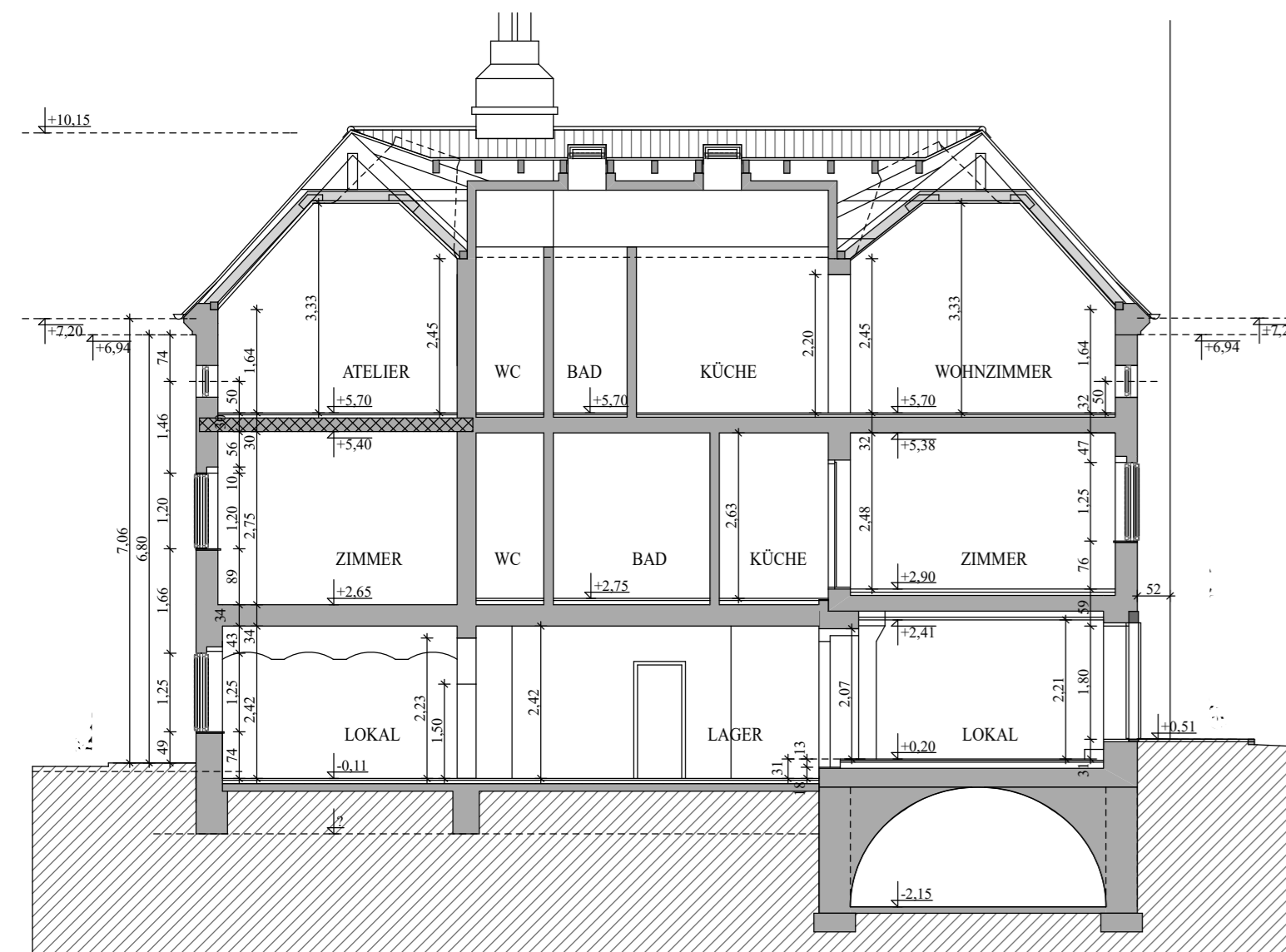
SCHNITT A-A 1:100
